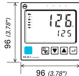
Frontansicht KS42-1
